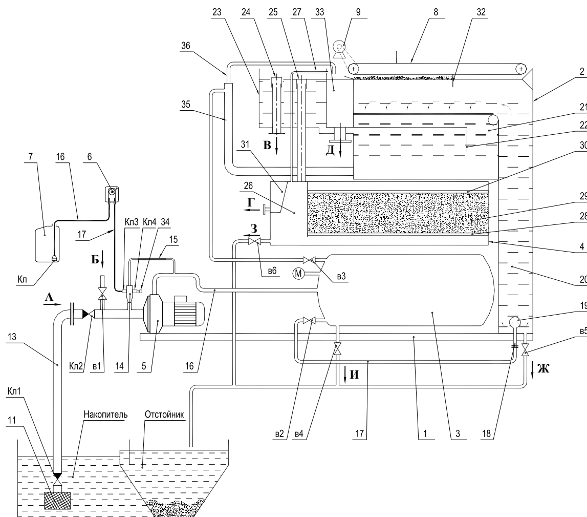
Рис.2. Технологическая схема установки ФФУ-10
